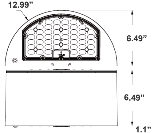
12.99" (W) x 6.49" (H) x 6.49" (D)
